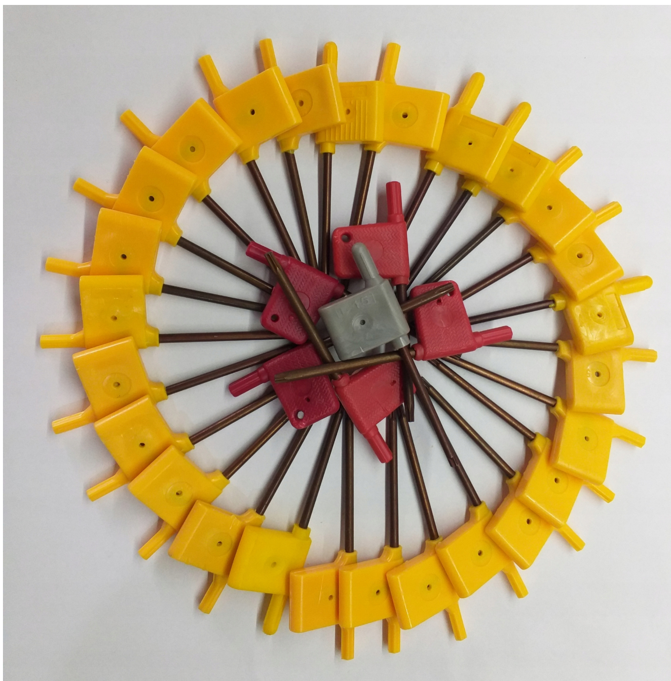
Klucz T15 torx do głowic/noży tokarskich
